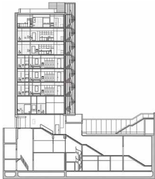
τομή ΕΕ
