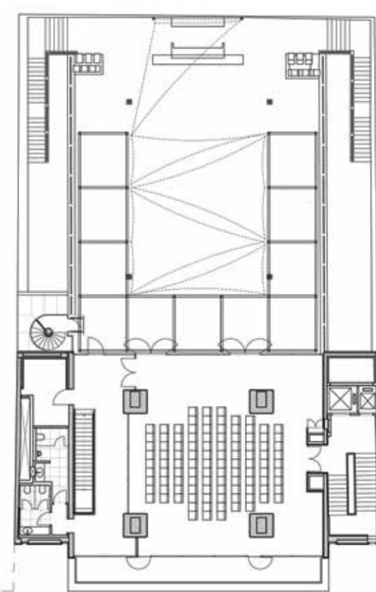
κάτοψη 1ου ορόφου
