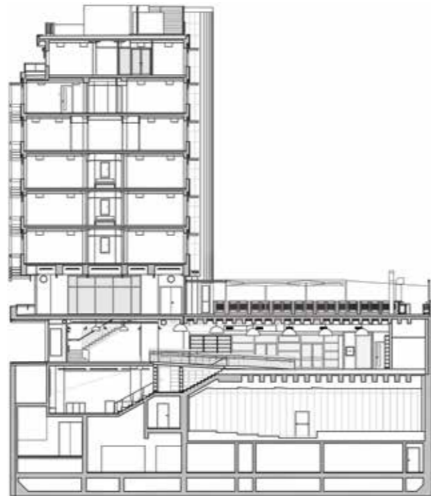
τομή ΒΒ
