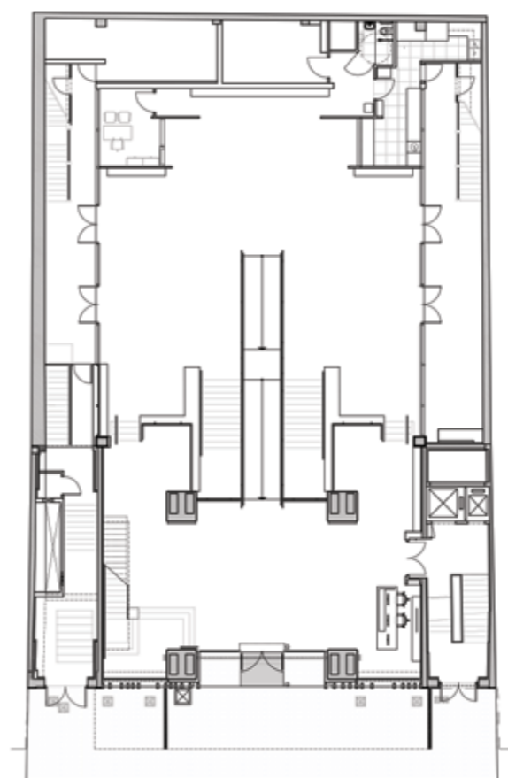
κάτοψη ισογείου
